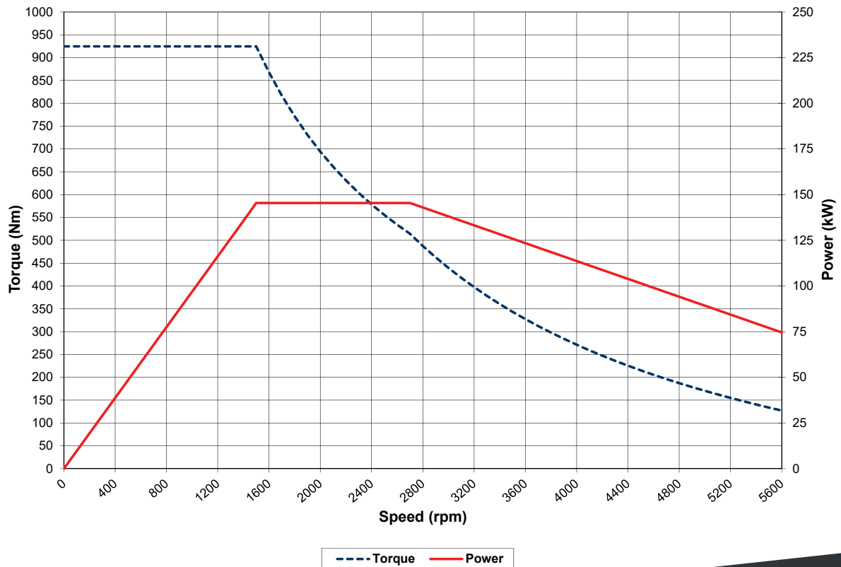
DA195 (S.I.)
